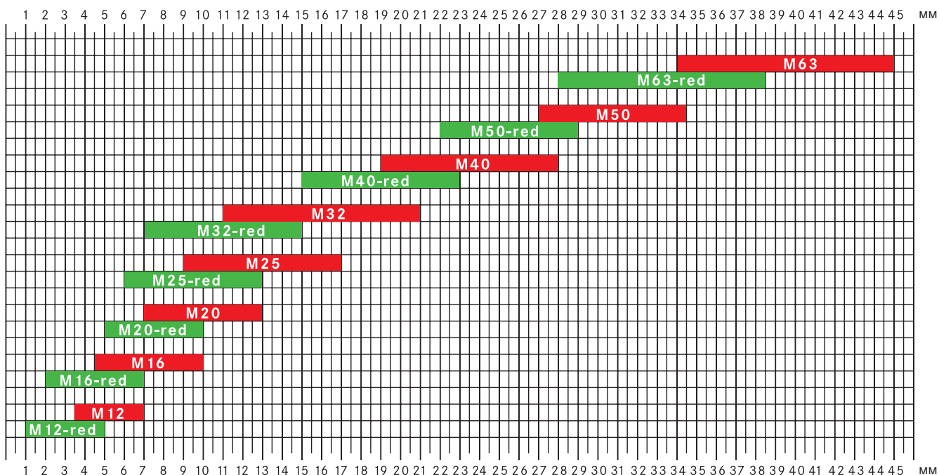
Диапазон фиксации метрической соединительной резьбы SKINTOP® SKINTOP® ST-M и SKINTOP® STR-M
