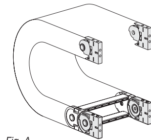
Fig. A Fissaggio della catena frontale, esterno/interno raggio. (Fig A) Vedi varianti di montaggio a pag. 31.
